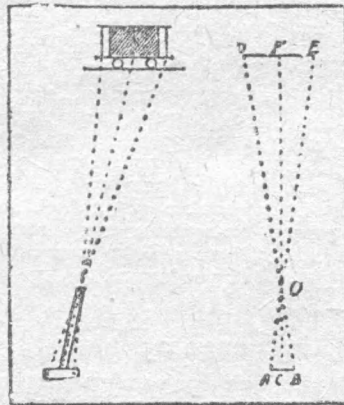
Рис. 4. Простейший дальномер и его употребление
