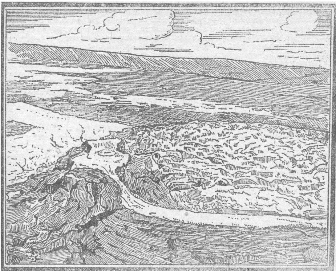
Рис. 3. Один из кратеров сопки Андрусова в Буманаской группе. Справа от кратера твердая высохшая корка. На переднем плане излившийся из кратера поток свежей грязи; еще ближе не затвердевшая, но уже разбитая трещинами кора; сзади—застывший поток, покрытый белыми выцветами солей
