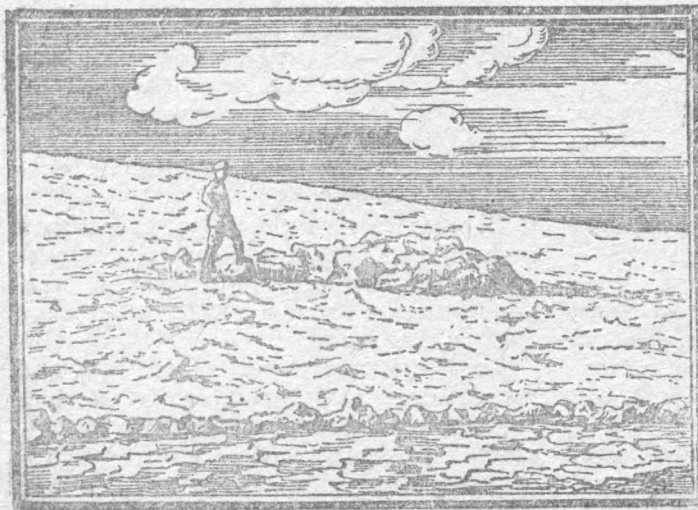
Рис. 4. Лавовое поле на Карапетовой горе, на месте извержения, бывшего весной 1929 года
